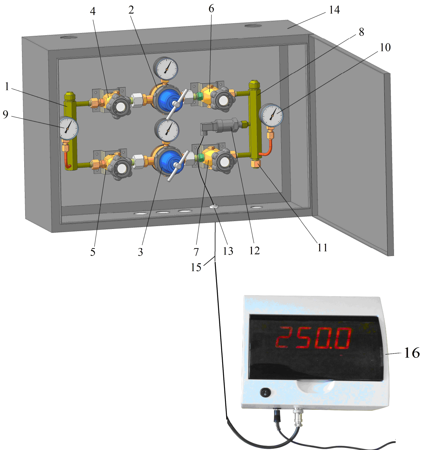
Рис. 1. Пост газопитания ПГК-10-100/10-100 с устройством СДКД
